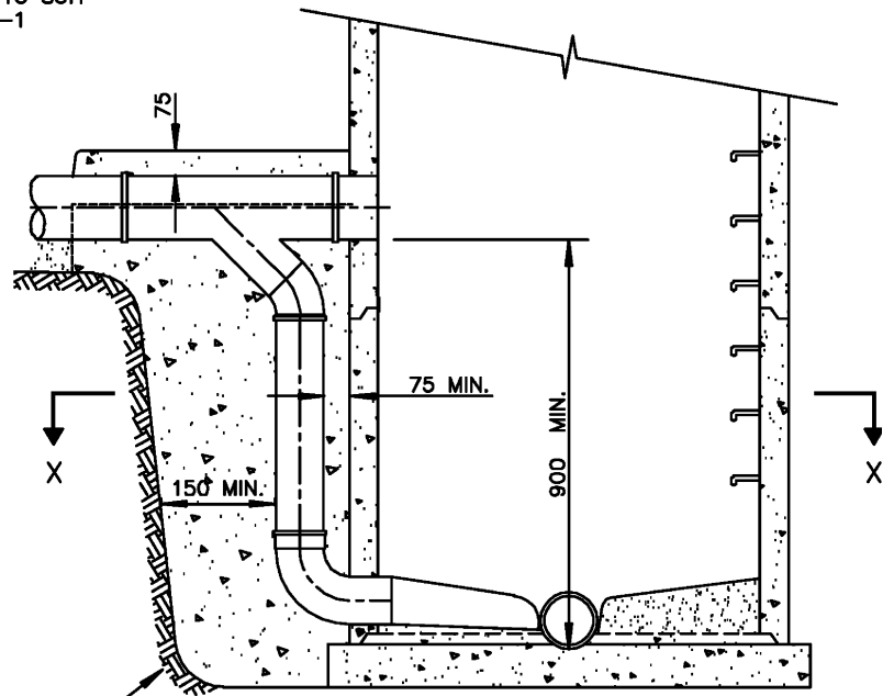
SECTION A-A DROP MANHOLE - TYPE I
