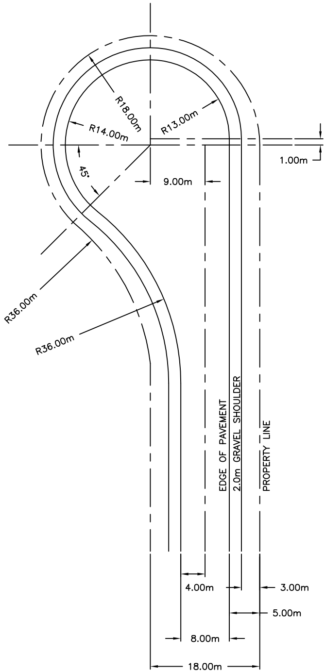
OFFSET CUL-DE-SAC
